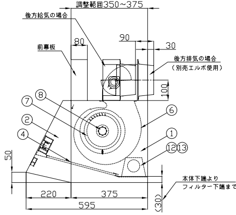
背面取付図
