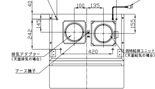
4-φ12ノックアウト (天吊用)
