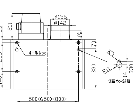
背面取付図
