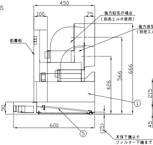
背面取付図
