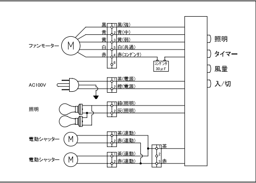
□ 結線図
