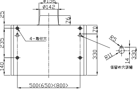
背面取付図
