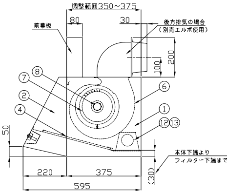
背面取付図
