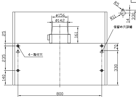
背面取付図
