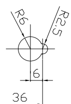
仮留め穴詳細
