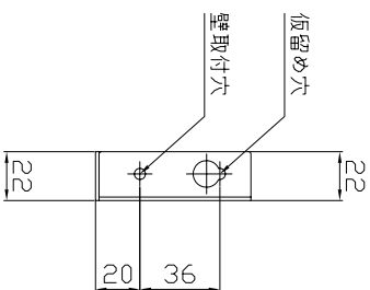
仮留め穴詳細
